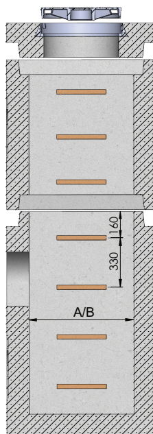
מכסה קוטר 50/60 ס"מ
