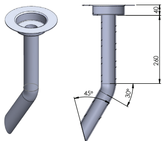
נקז ריצפה תת אספלט זוויתי קטרים: לפי דרישה
