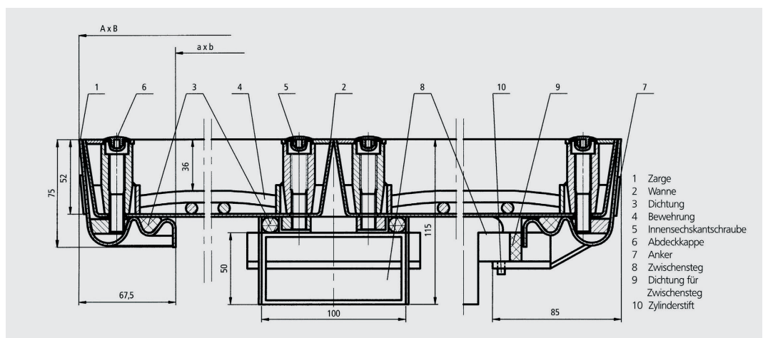
פלדה BV-RA / פלדת אל חלד BE-RA, קנה מידה: 1:2.5
