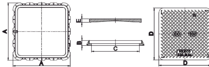
KIO SQUARE B125 CLASS
