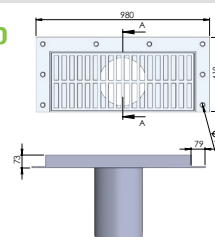
חומר: פלדה מגולוונת עומס: D400
